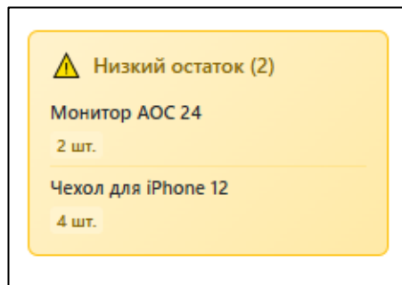
Рисунок 2.9 – Вид уведомления
