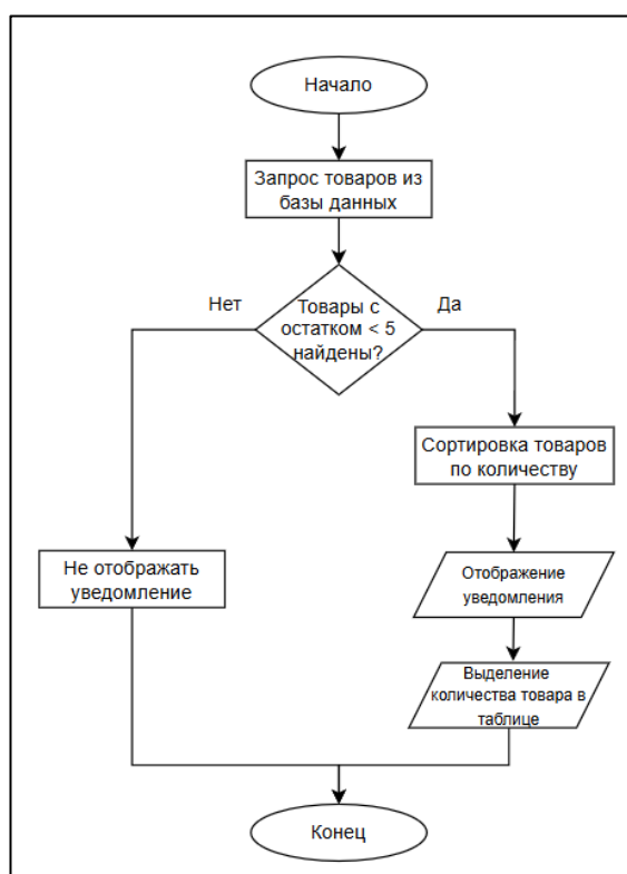
Рисунок 2.5 – Блок-схема уведомлений
