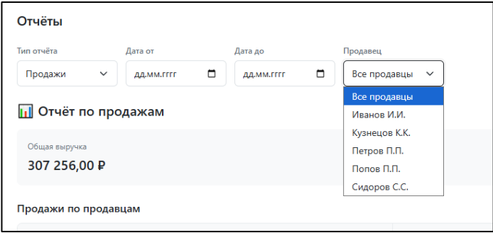
Рисунок 2.12 – Сортировка отчётов
