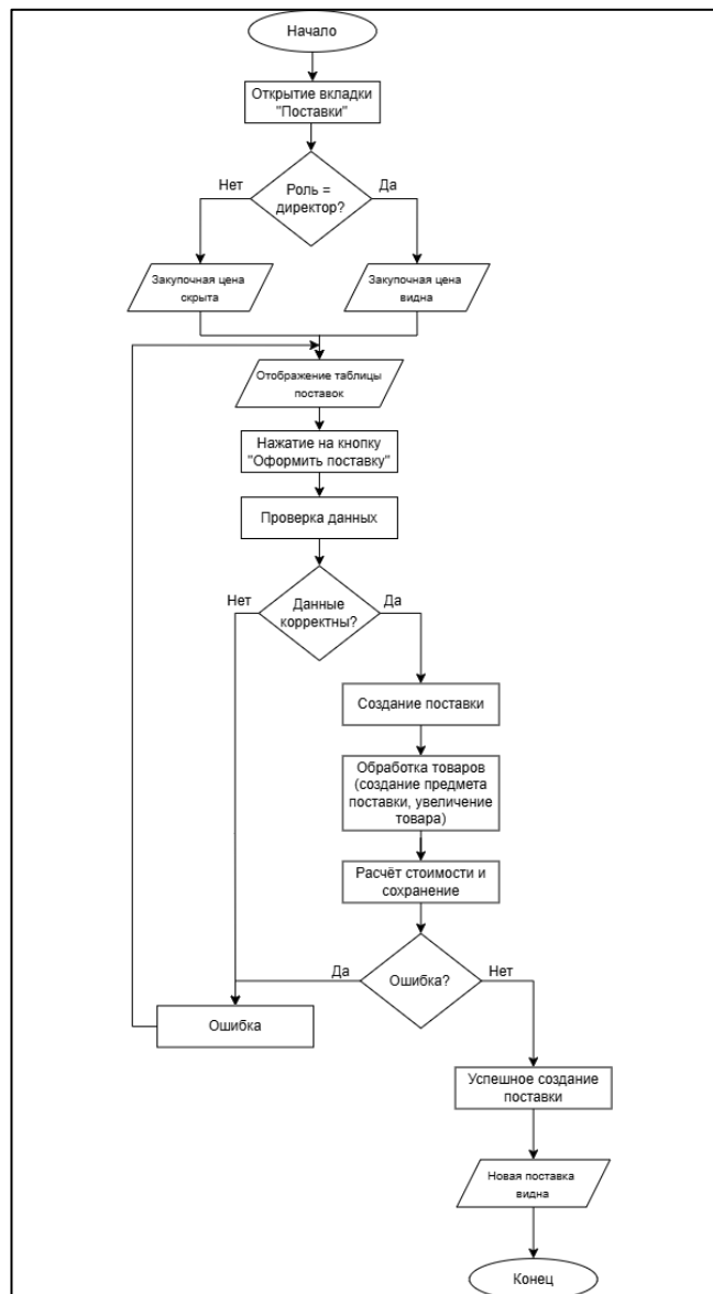
Рисунок 2.7 – Блок-схема поставок
