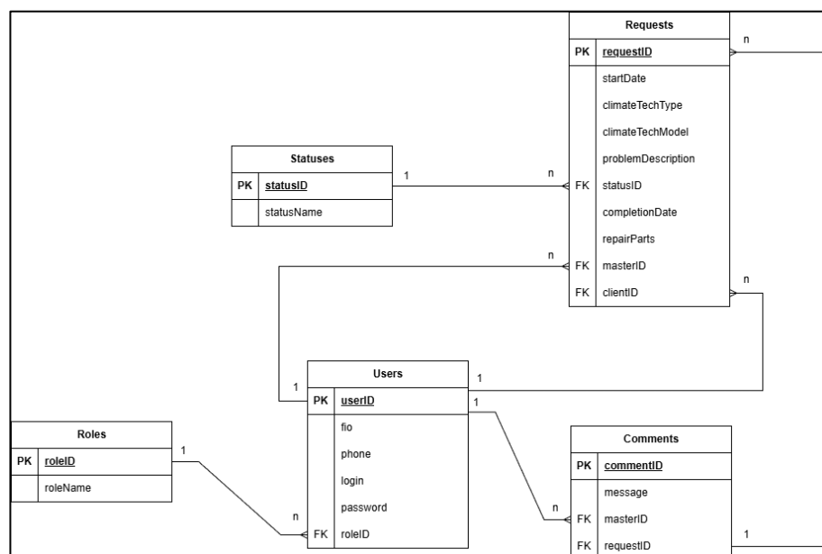
Рисунок 1.1 – ERD-диаграмма
